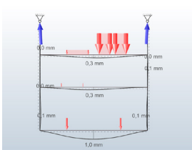
Statikai rendszer
