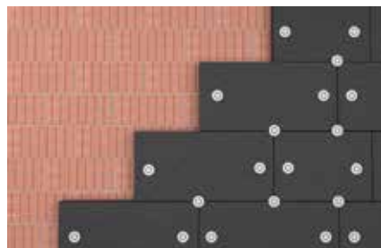
Polisztirol szigetelőtábla rögzítése
